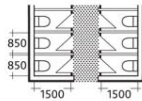
WC-Kabinen, 2-bündig angeordnet
