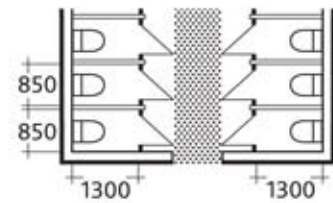
WC-Kabinen, 2-bündig angeordnet
