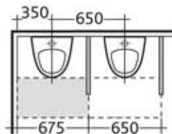
nebeneinander zur Wandecke mit Trennwänden
