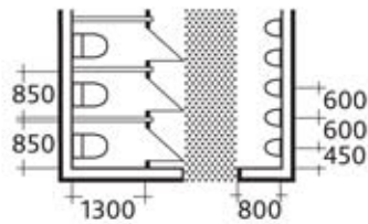
WC-Kabinen mit gegenüberliegenden Einzelurinalen
