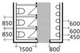
WC-Kabinen mit gegenüberliegenden Einzelurinalen
