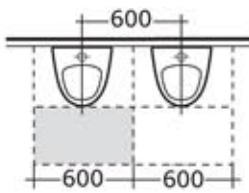
nebeneinander auf ebener Wand
