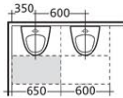
nebeneinander zur Wandecke
